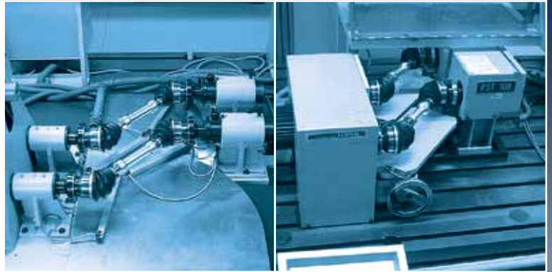
Système d'étanchéité TPE de l'arbre de transmission pour les joints AAR
