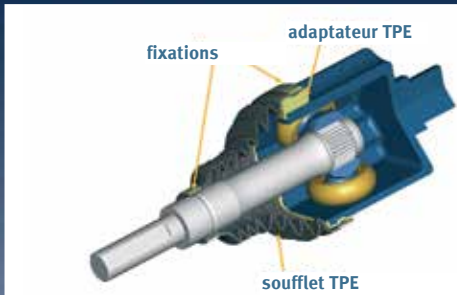
Système d'étanchéité TPE de l'arbre de transmission pour les joints AAR
